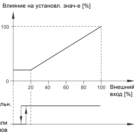
Рис. 38 "Линейно с остановом" и "Линейно с мин."
