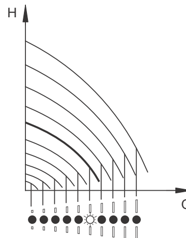
Рис. 17 Насос в режиме управления с постоянной характеристикой
