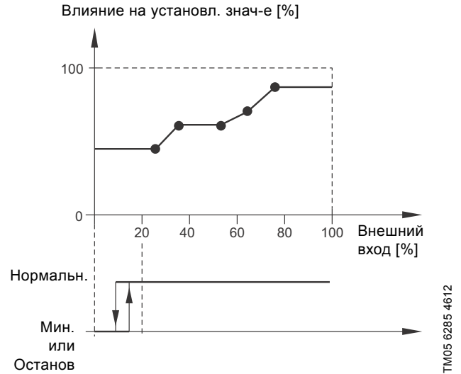
Рис. 42 Таблица влиян. с остан. у мин.
