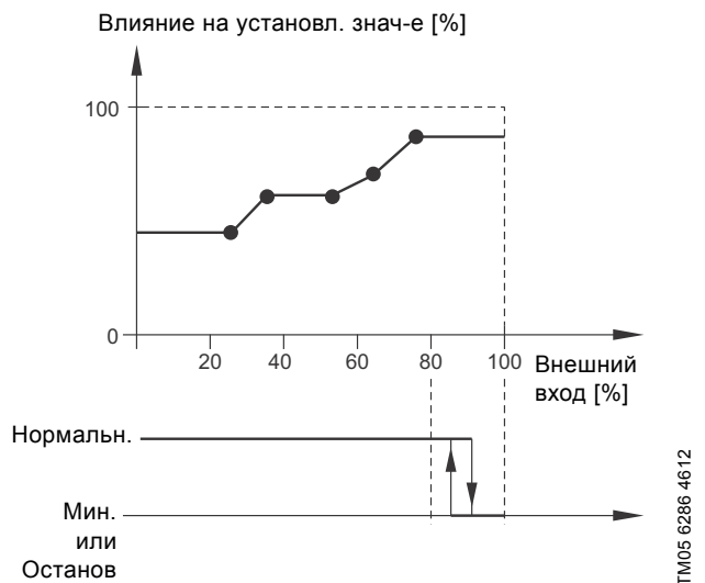
Рис. 43 Таблица влиян. с остан. у макс.
