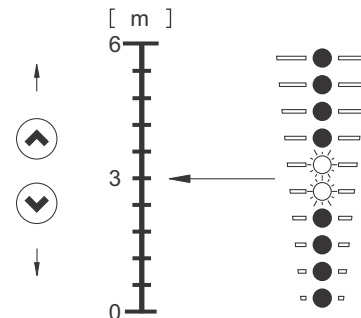
Рис. 16 Заданное значение 3 м, управление перепадом давления
